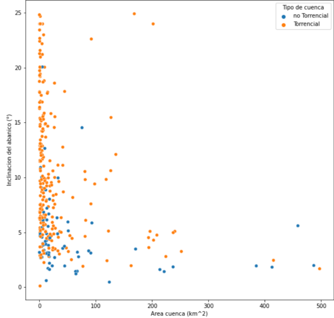
Inclinación abanico vs Área cuenca
