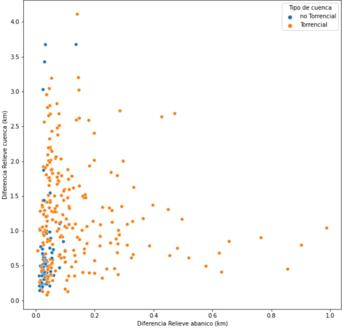
Diferencia relieve abanico vs diferencia relieve cuenca
