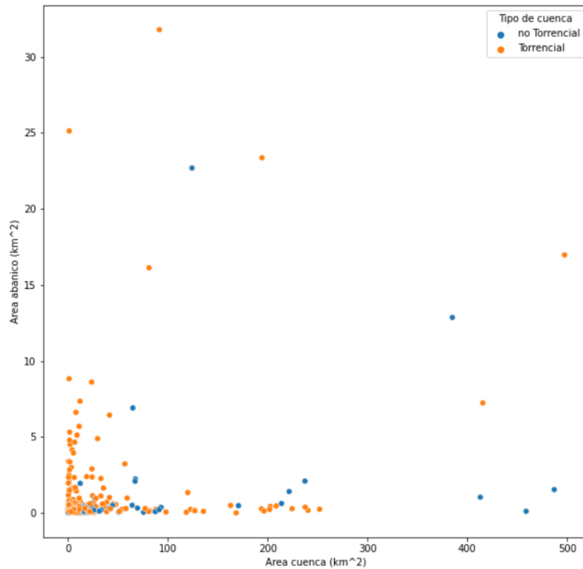
Área cuenca vs área abanico
