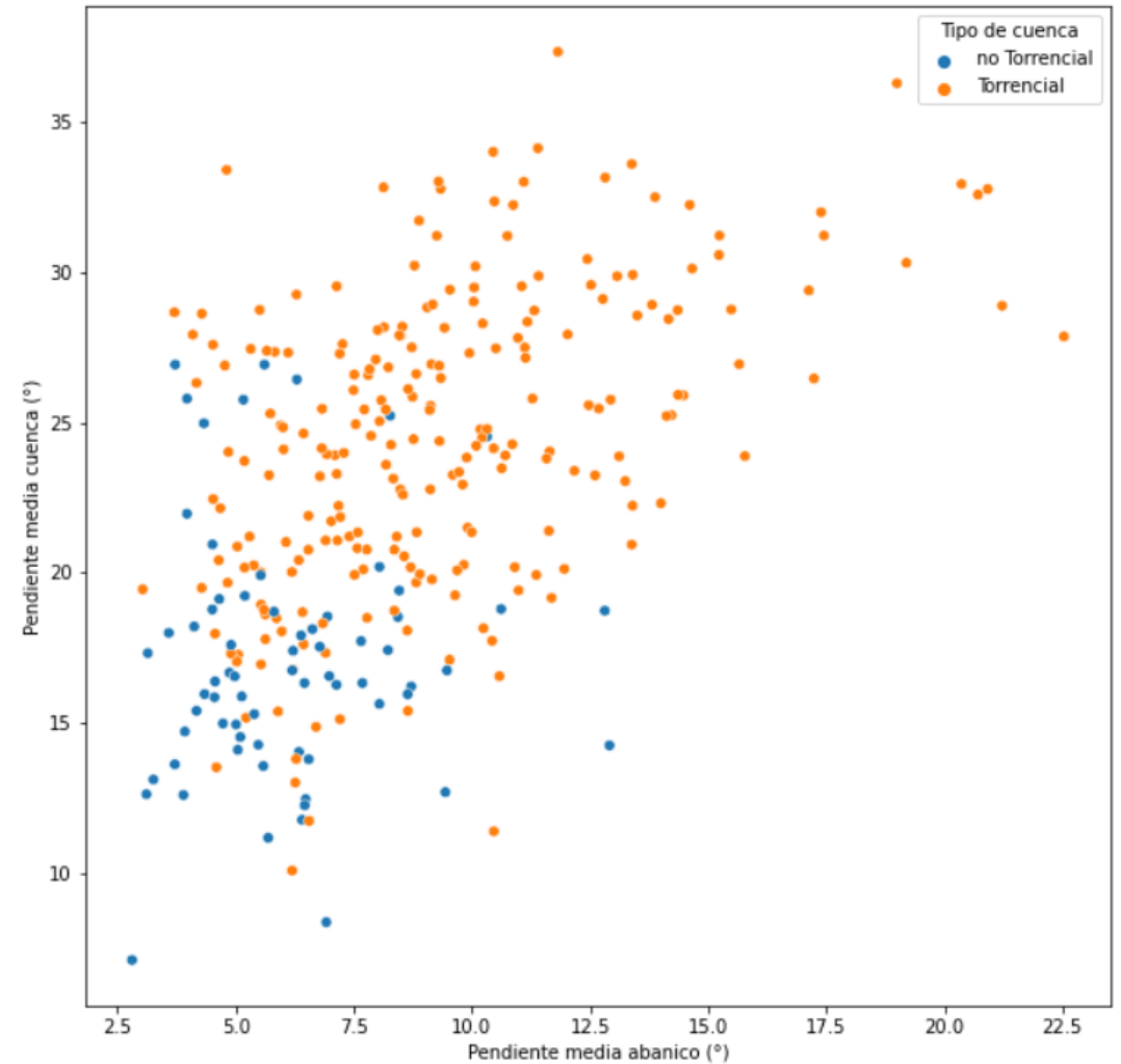
Pendiente cuenca vs pendiente abanico
