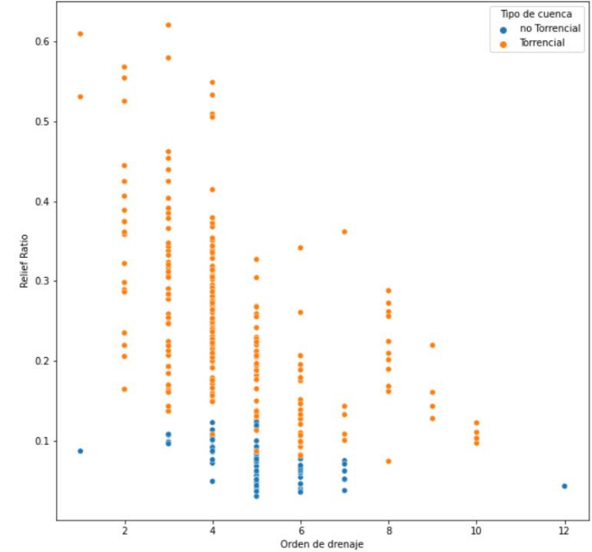
Clasificación, según Aristizábal & Gómez, 2020
