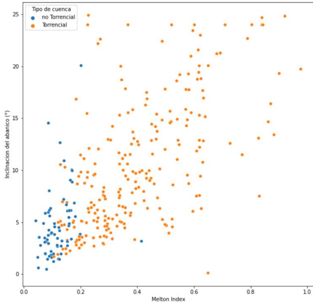
Inclinación abanico vs Melton índice
