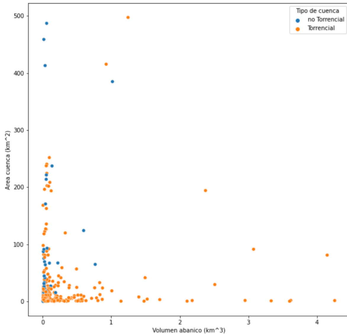
Área cuenca vs Volumen abanico
