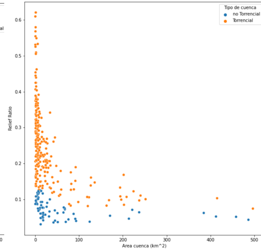
Clasificación, según Aristizábal & Gómez, 2020
